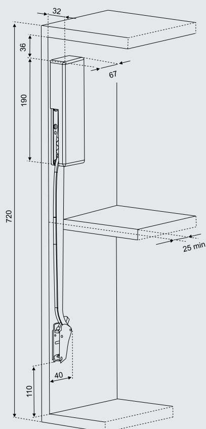
Габаритные размеры системы.
